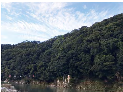
写真2 相模川の谷
