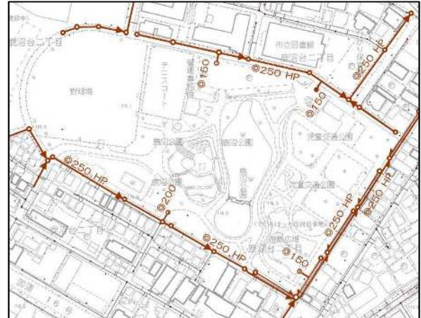
< 鹿沼公園周辺の汚水管理設図 >
