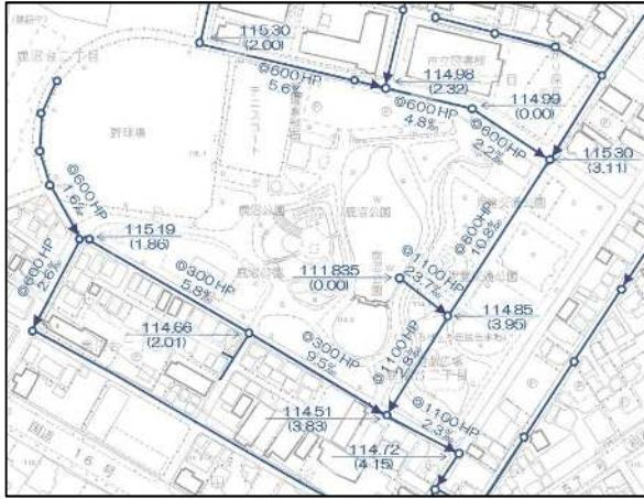
< 鹿沼公園周辺の雨水管理設図 >
