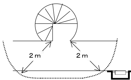
屋外避難階段の周囲 2 m の範囲
