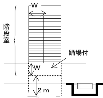
階段を出た正面 2 m の範囲
