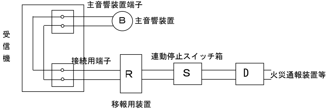
移報用装置 第 12-36 図
