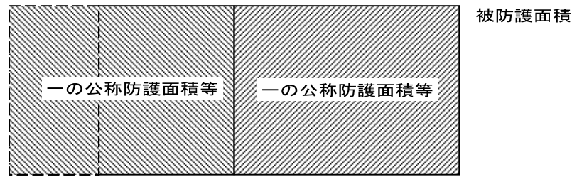
第 25-9 図 防護対象物が大きく一の装置で警戒できない場合
