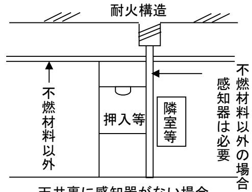
天井裏に感知器がない場合 第 12—7 図
