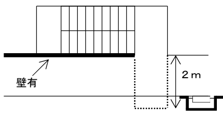
屋外階段の正面 2 m の範囲
