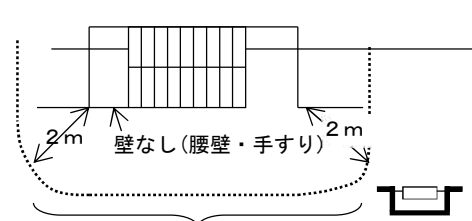
屋外避難階段の周囲 2 m の範囲
