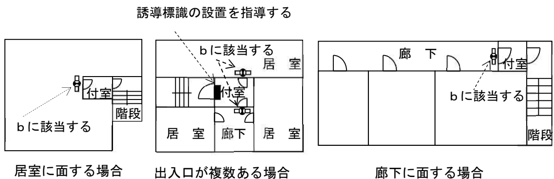
第18-14図 直通階段の出入口の例
