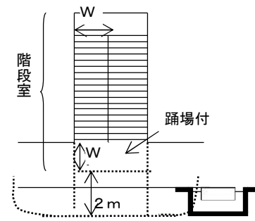
屋外避難階段を出た正面 2 m の範囲
