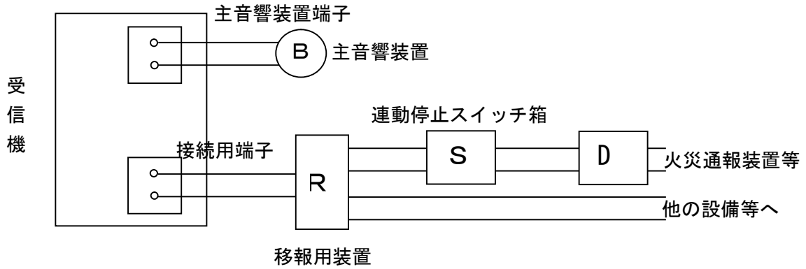
移報用装置 第 12-35 図
