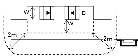
屋外避難階段を出た正面 2 m の範囲
