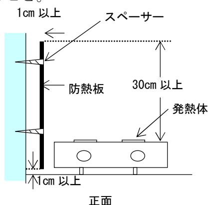
第4-1図 防熱板の設置例1（発熱体が露出）
