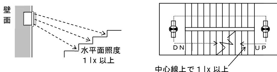
第 18-31 図 階段通路誘導灯の設置例
